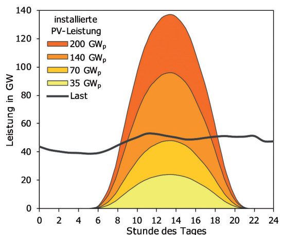
Abbildung 1: Elektrische Last und PV-Erzeugung bei unterschiedlichen Ausbauszenarien an einem Sonntag in Deutschland [Daten 21.07.2013: PV-Erzeugung bei 35 GW p (EEX), Last (ENTSO-E)].
