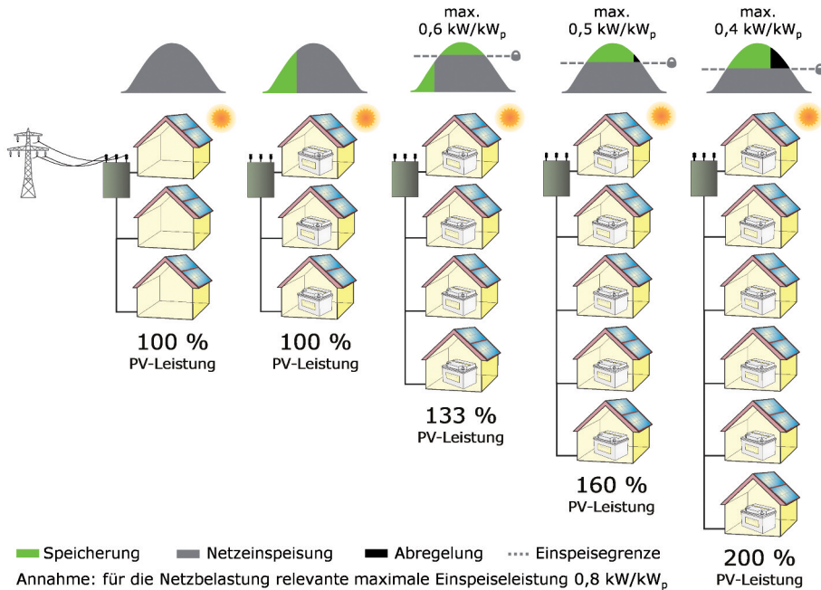
Abbildung 4: Einfluss der Betriebsstrategie und Einspeisegrenze auf die maximale Aufnahmefähigkeit der Netze im Verhältnis zum maximalen PV-Ausbau ohne Einspeisebegrenzung [1]
