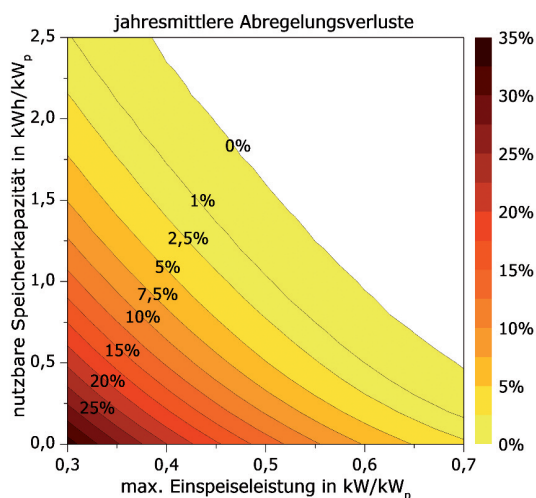
Abbildung 3: Typische jährliche Abregelungsverluste von PV-Systemen mit Speicher in Abhängigkeit der maximalen Einspeiseleistung und nutzbaren Speicherkapazität [2] (Annahmen: kein Eigenverbrauch durch die Last am Tag, Speicherladung ausschließlich mit Energie oberhalb der jeweiligen Einspeisegrenze, vollständige Speicherentladung in der Nacht).
